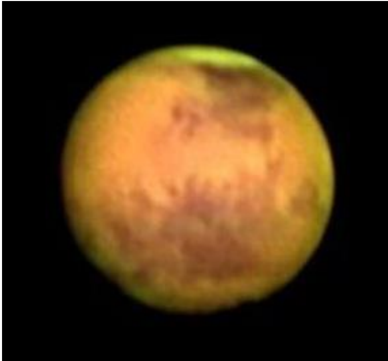
Mars (08.01.2008)
